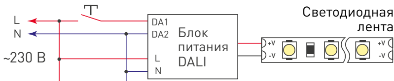
Рис. 1. Схема подключения при использовании внешней кнопки (Push DIM).
