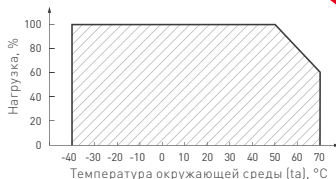
Рис. 3. Максимальная допустимая нагрузка, % от мощности источника.
